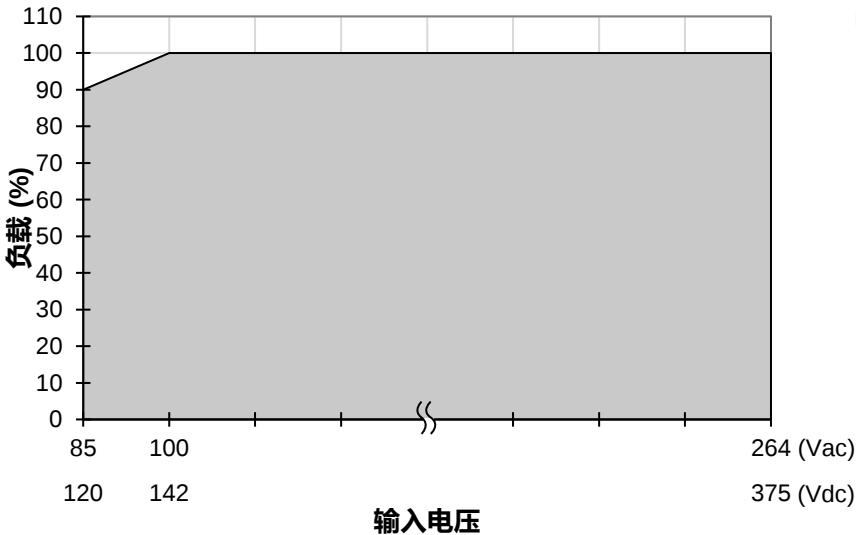
图. 2 AC 输入电压功率降额 < 100 Vac 功率降额 1 % / Vac < 142 Vdc 功率降额 1 % / Vdc
