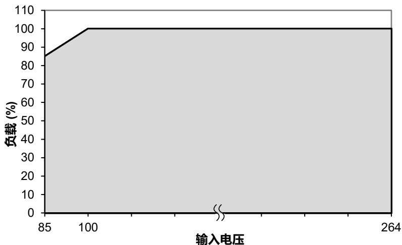
图. 2 AC 输入电压功率降额
