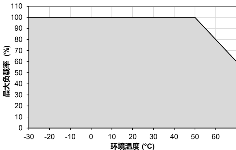
图.1 垂直安装功率降额
