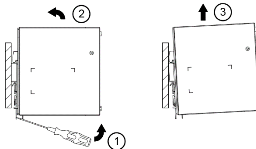
图. 3.2 拆卸
