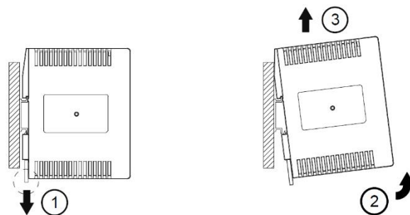
图. 2.2 拆卸
