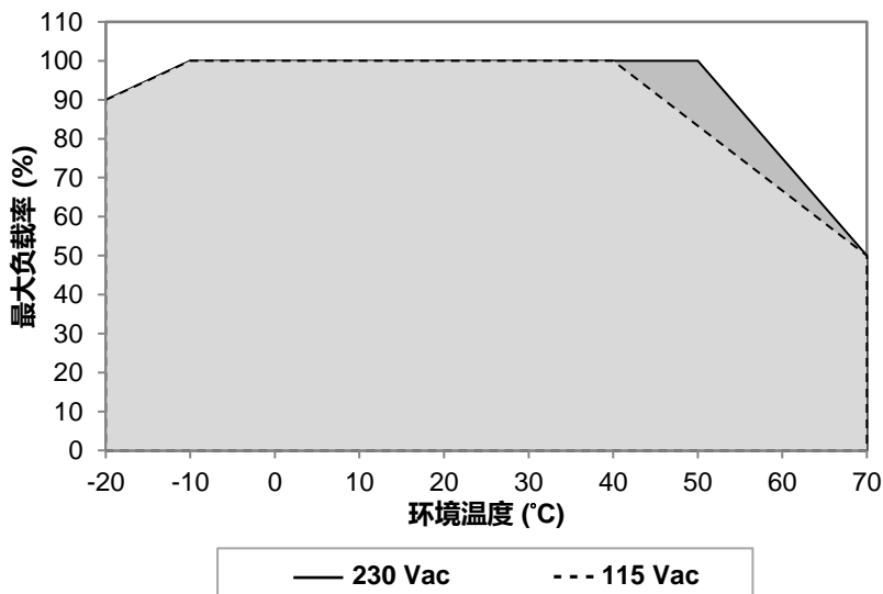
图. 1 功率降额, 垂直安装
