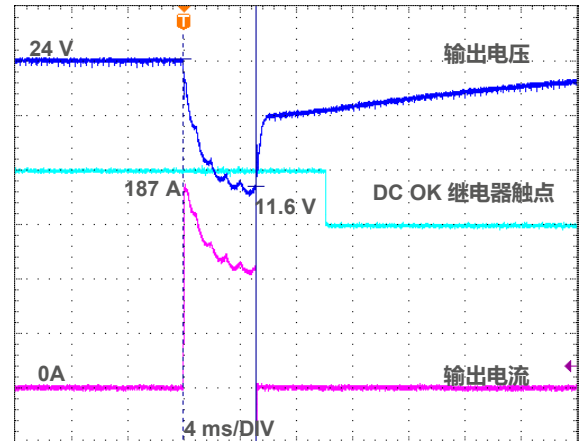
图 8.4 APB 500% 额定输出电流, 持续 5 ms
