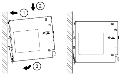
图. 6.1 安装
