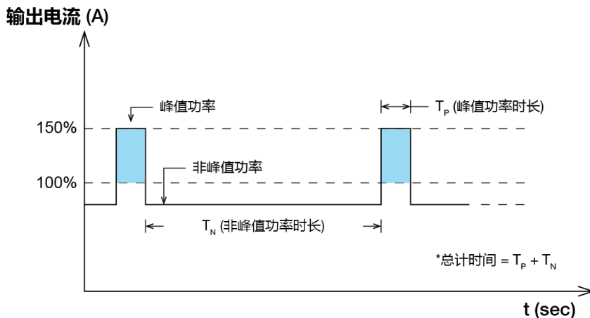
图. 7 占空比计算
