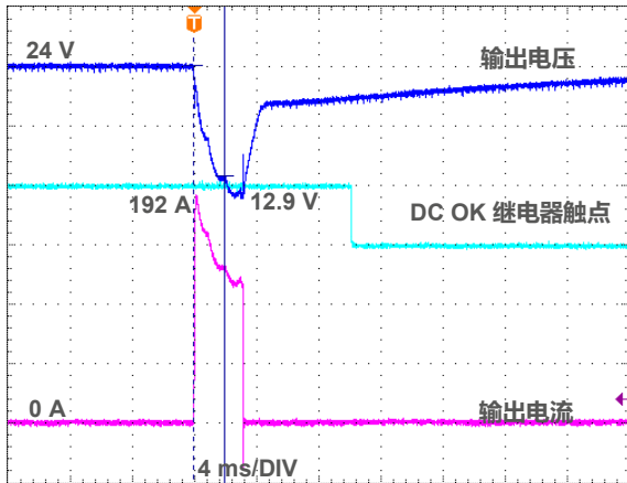
图 8.3 APB 500% 额定输出电流, 持续 2 ms
