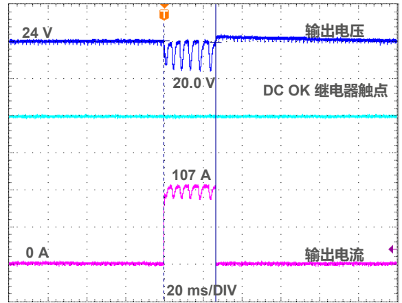
图 8.2 APB 275% 额定输出电流, 持续 25 ms
