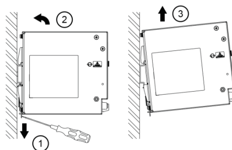
图. 6.2 拆卸
