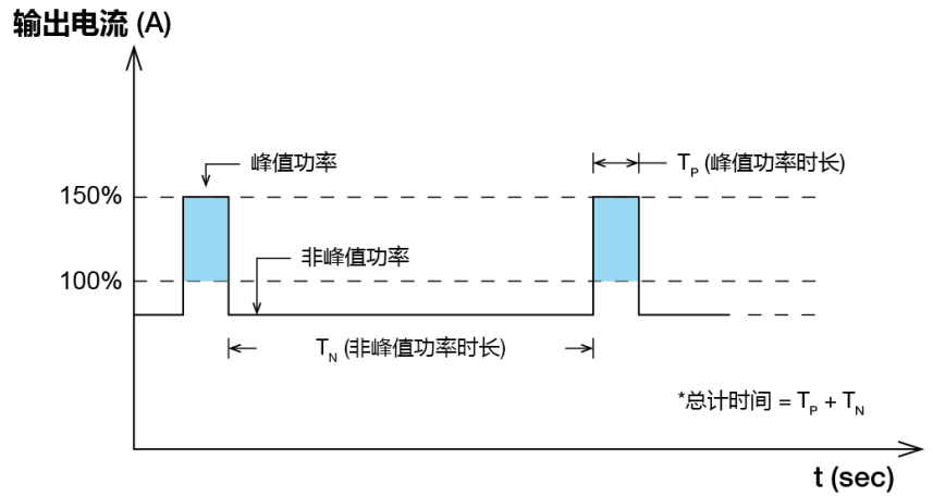
图. 7 占空比计算
