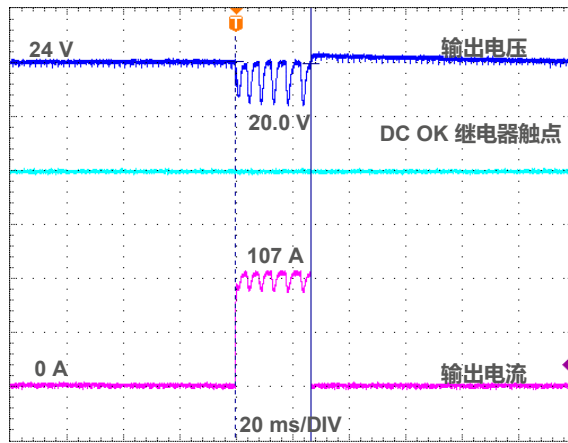
图 8.2 APB 275% 额定输出电流, 持续 25 ms
