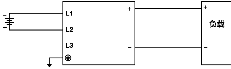
图. 12 DC 输入接线示意图
