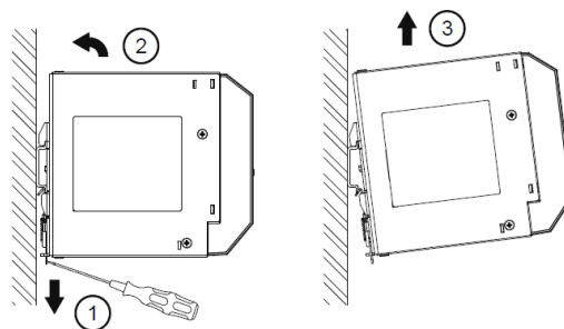
图. 6.2 拆卸
