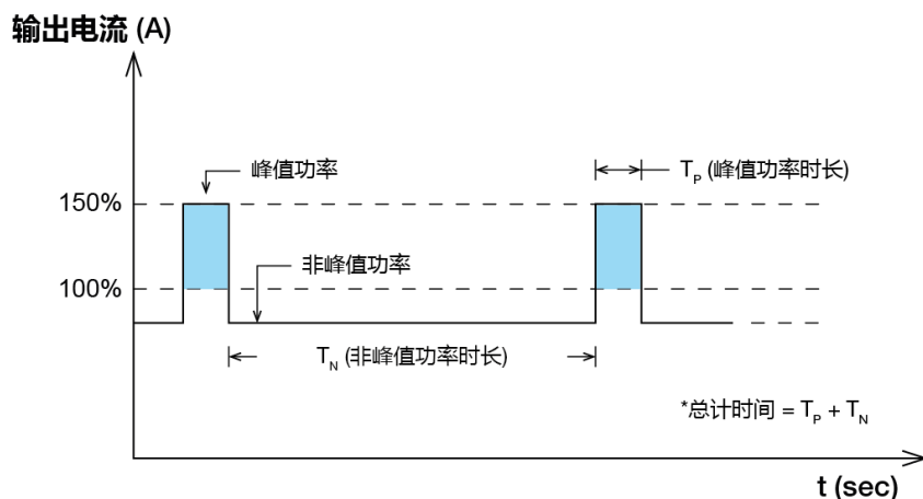
图. 7 占空比计算
