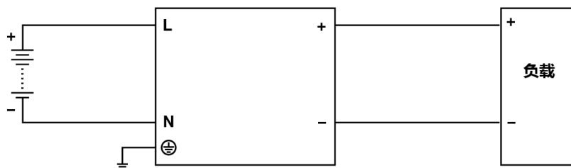
图. 12 直流输入模式连接电路图
