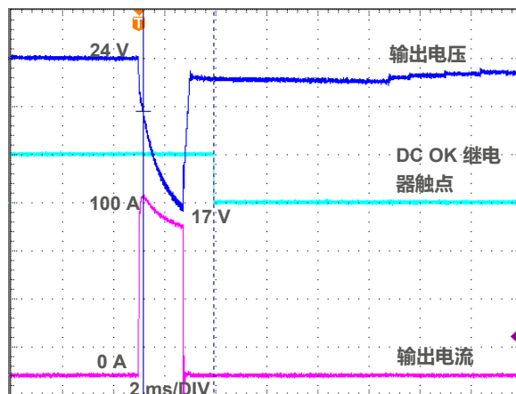
图. 8.2 APB 500%额定输出电流持续 2 ms
