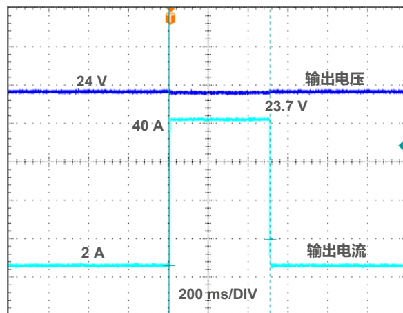
图. 8.4 APB 200%额定输出电流持续 500 ms
