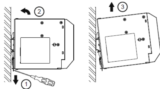
图. 6.2 拆卸
