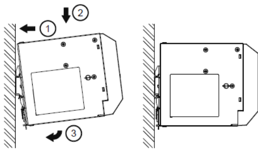
图. 6.1 安装
