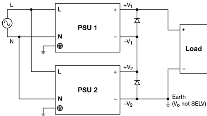
图. 11 串联模式连接电路图
