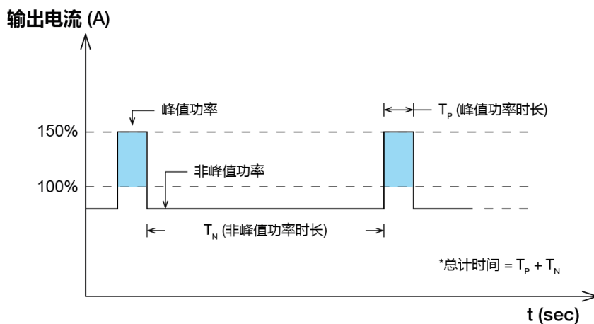
图. 7 占空比计算
