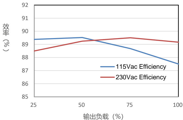
图 1-1 MEA-065A12C 效率对比输出负载
