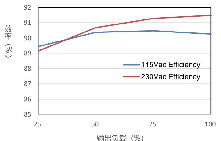
图 1-4 MEA-065A24C 效率对比输出负载
