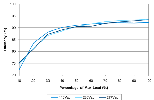
LNE-48V100W□
