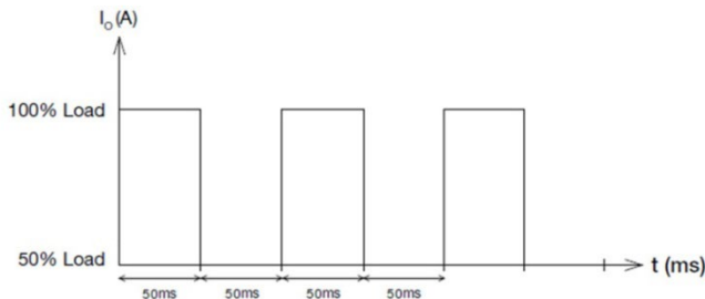
Fig. 5 Dynamic Load
