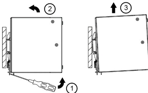
图. 3.2 拆卸
