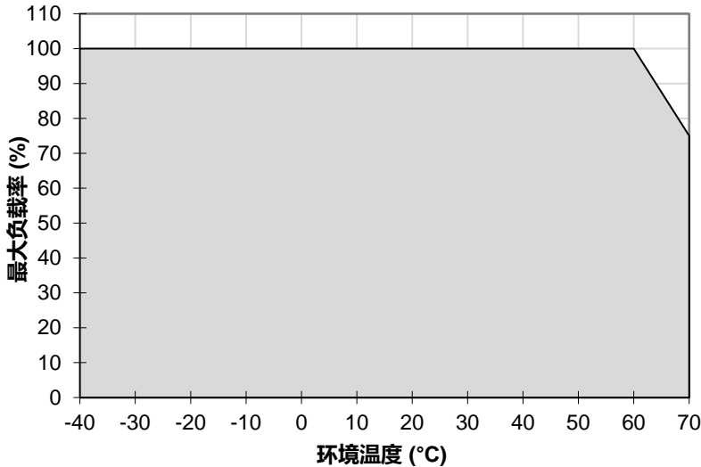
图. 1 垂直安装降额 > 60°C 功率降额 2.5% / °C
