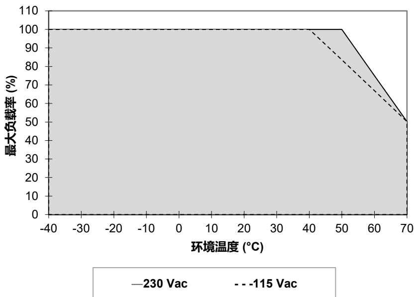
图. 1 垂直安装降额
