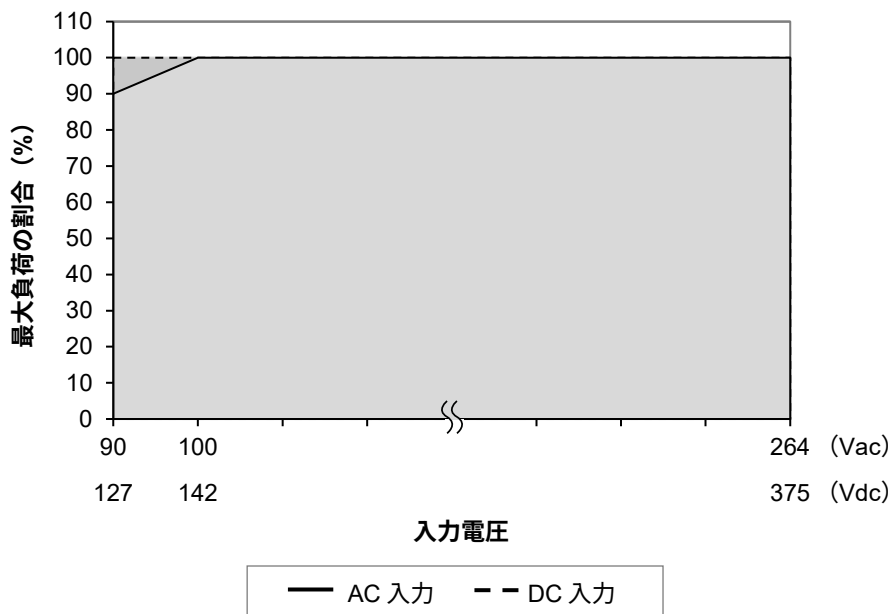
図2 ACおよびDC入力電圧の定格低減 < 100 Vac 電力を 1%低減 / Vac DC入力の電力定格低減なし
