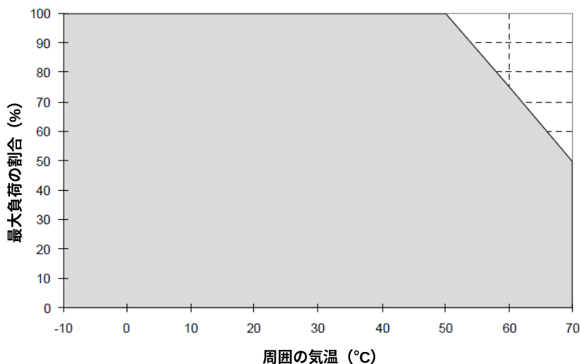
図 1 垂直マウント時の定格低減
