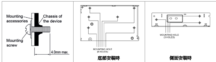
图四. 安装螺丝
