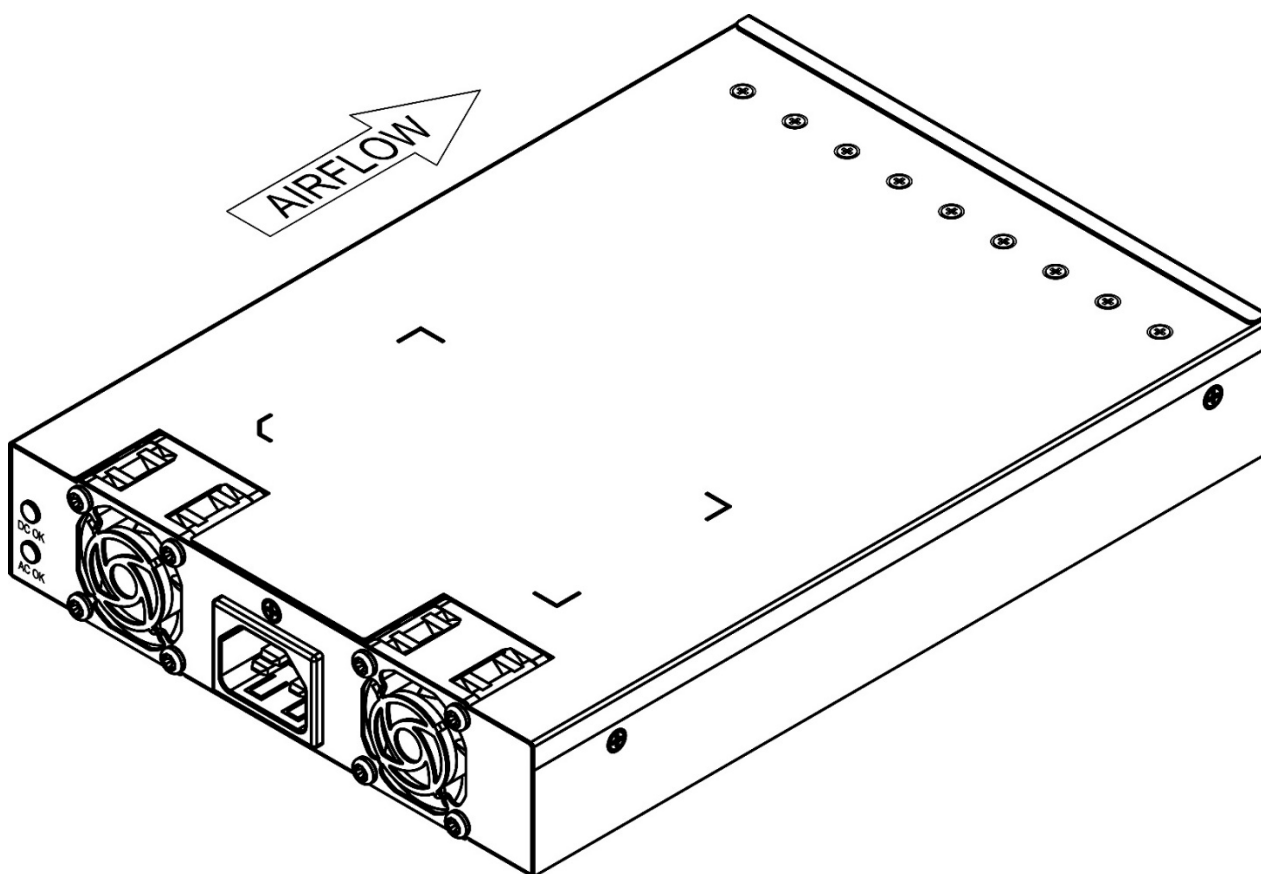
Fig. 1: MEG-3K0A series
