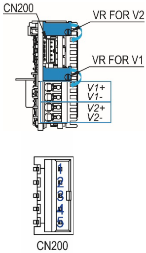
Fig. 17: -x3 Module connector
