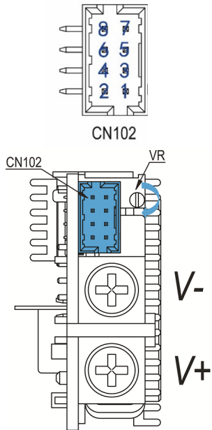
Fig. 15: -x1 Module connector
